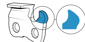
山型 デプスゲージ
